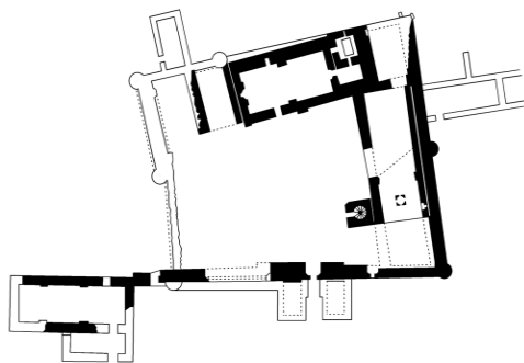
Рис. 4. Ханегя Пир-Хусейна (XI в.) на реке Пирсагат
